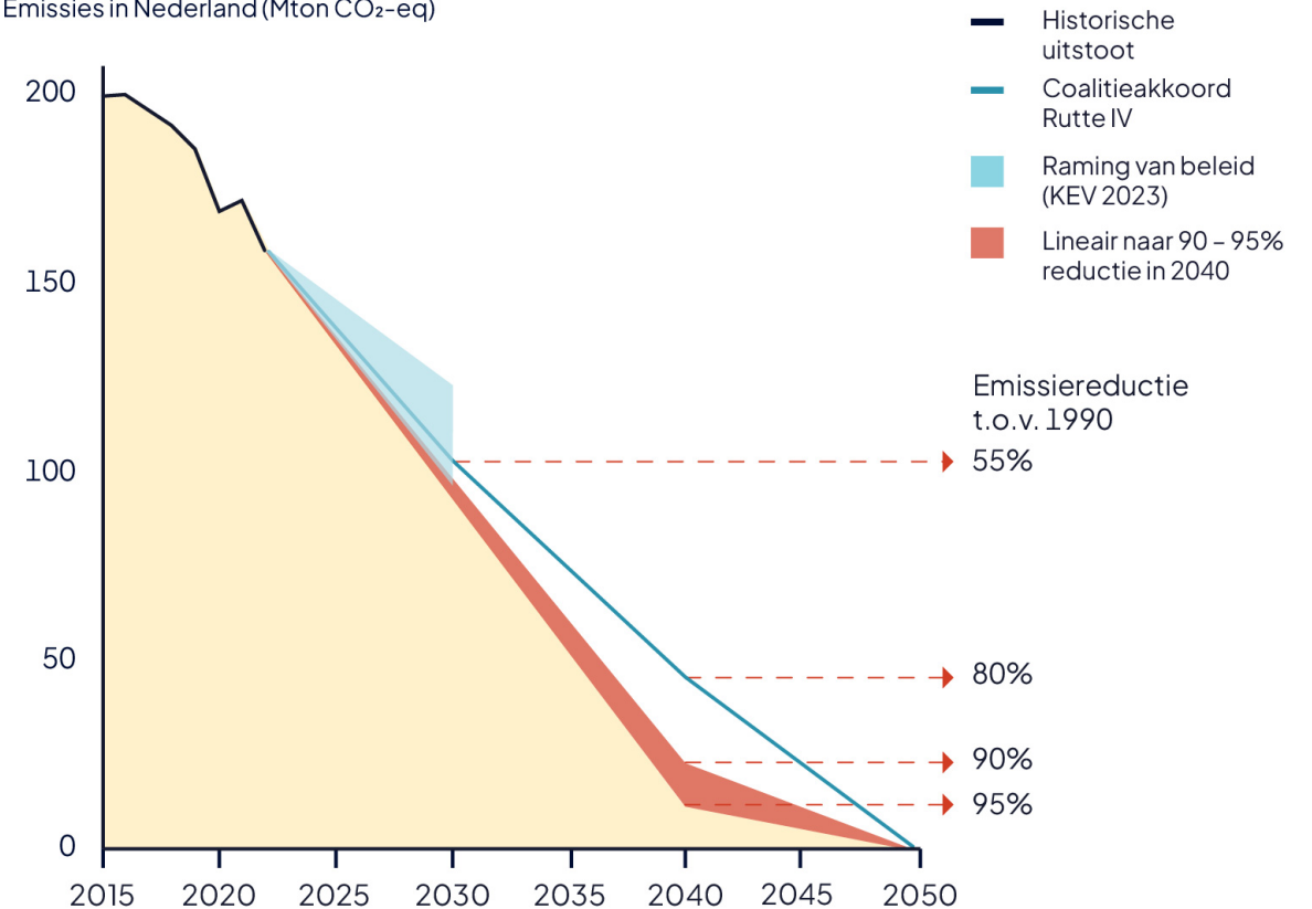
Emissies in Nederland (Mton CO 2 -eq)
